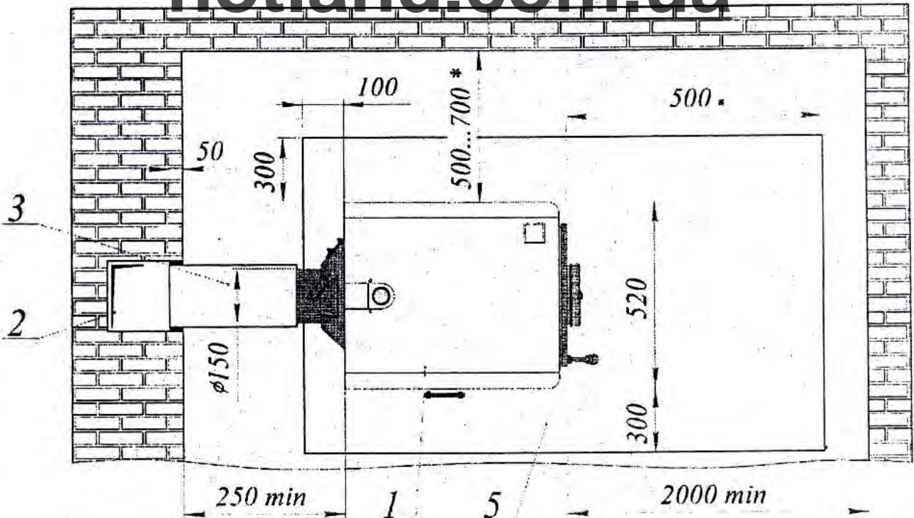
Рис. 2. Рекомендована схема установки котла і під'єднання до димової труби:
