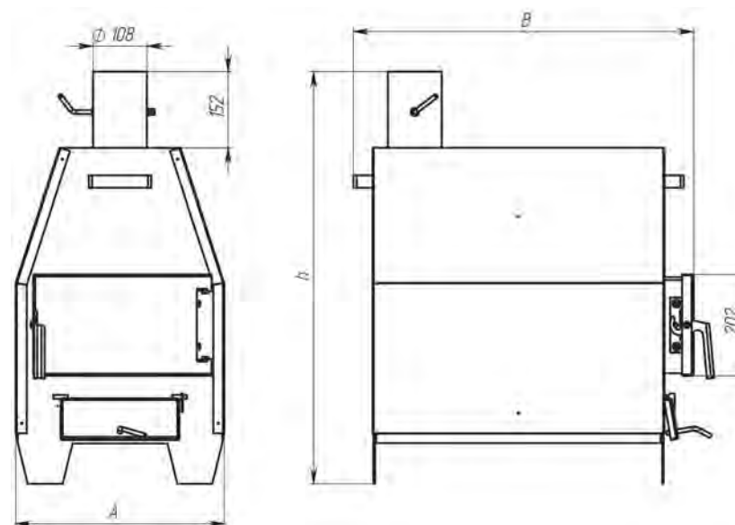
Габаритные и присоединительные размеры печи ПДГ «ZUBR»
