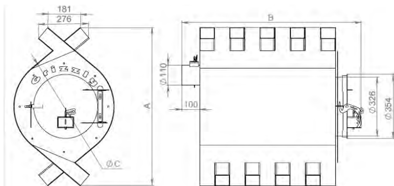
Приложение № 1 Габаритные и присоединительные размеры печи ПДГГ «GRIZZLY»
