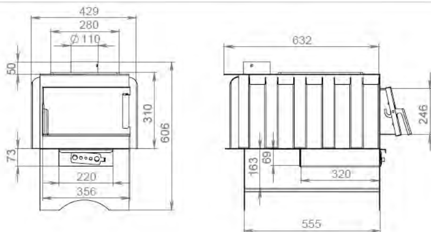
Габаритные и присоединительные размеры печи ПДГП «PANDA»
