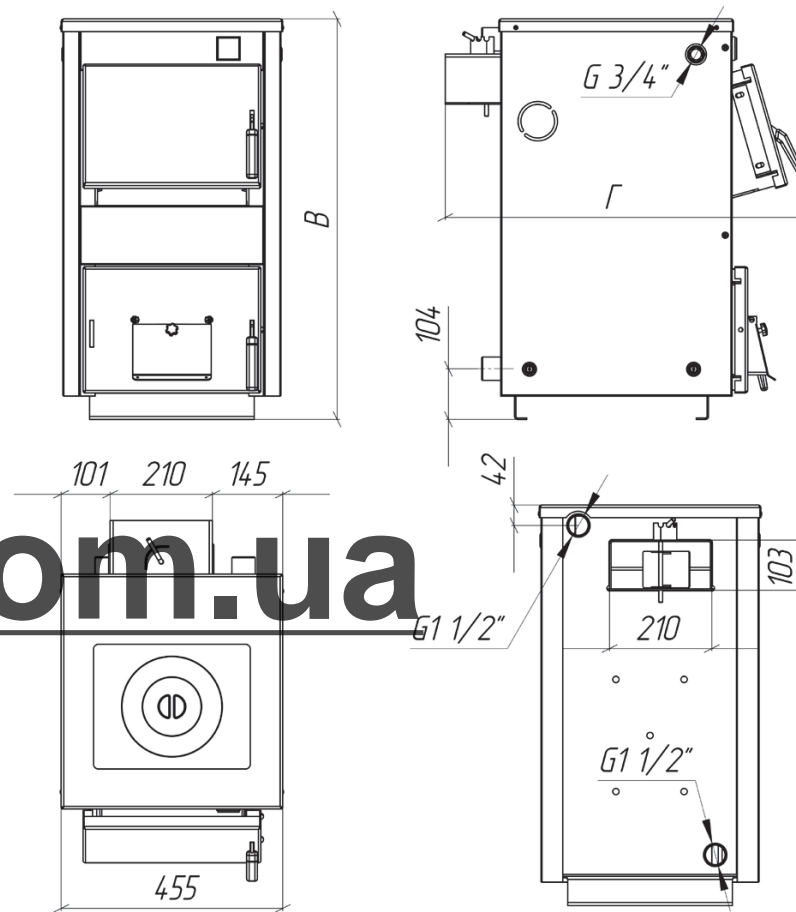
Габаритные и присоединительные размеры котлов ТП с
