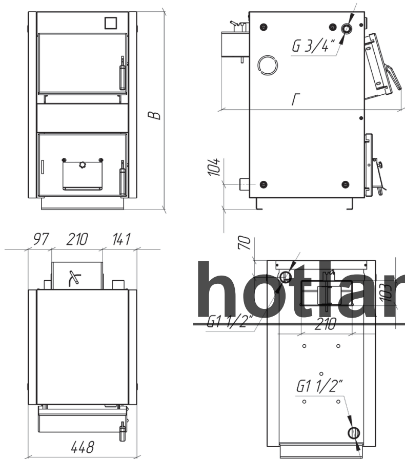
Габаритные и присоединительные размеры котлов ТТ с
